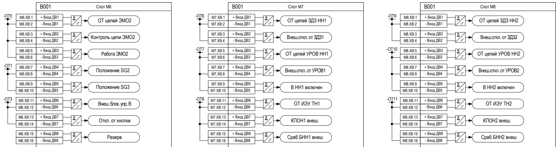
Рисунок Д.3 – Подключение дискретных входов и выходов к внутренним сигналам алгоритмов для блоков в слотах М6-М8
